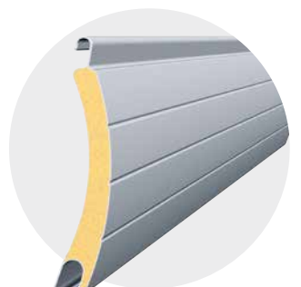
Aluminiumprofil A53
